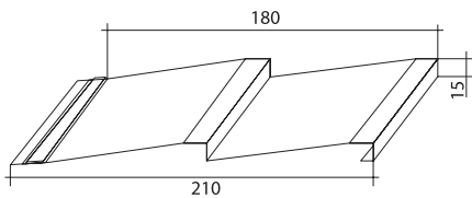
Двойная волна с ребром.
