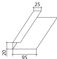
Крепежная планка
