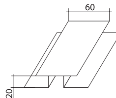
Нащельник
