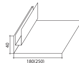
Откосная планка шириной 180 или 250 мм
