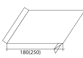
Водоотлив оконный шириной 180 или 250 мм
