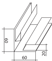
Угол наружный
