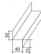
Верхний отлив
