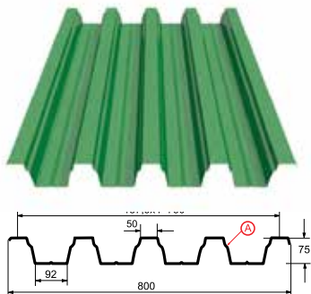
Профилированный лист H-75x750-A Толщина материала 0.65 - 1.0 мм
